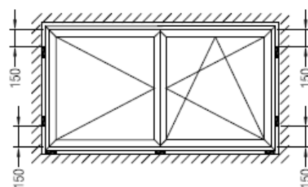
Dvoukřídlé okno s pohyblivým sloupkem (nosný blok v oblasti pohyblivého sloupku nesmí ovlivňovat funkci okna)
