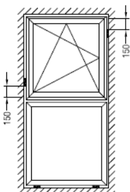
Jednokřídlé otvírávě - sklopné okno s pevným zasklením spodního nadsvětlíku (nosné bloky pod zasklívacími podložkami)
