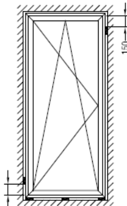
Balkonové dveře otvírávě - sklopné
